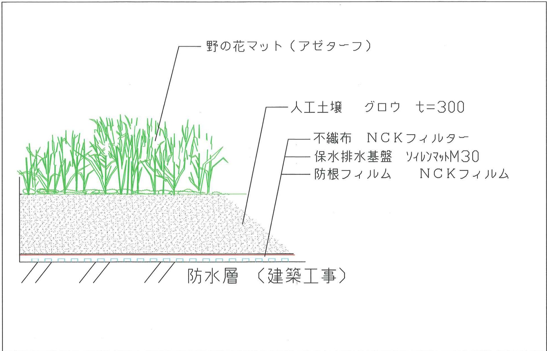
野の花マット（アゼターフ）断面図 日付 尺数 尺数
